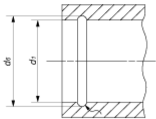
Форма В - для отверстий
