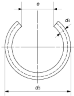
Форма А - для валов
